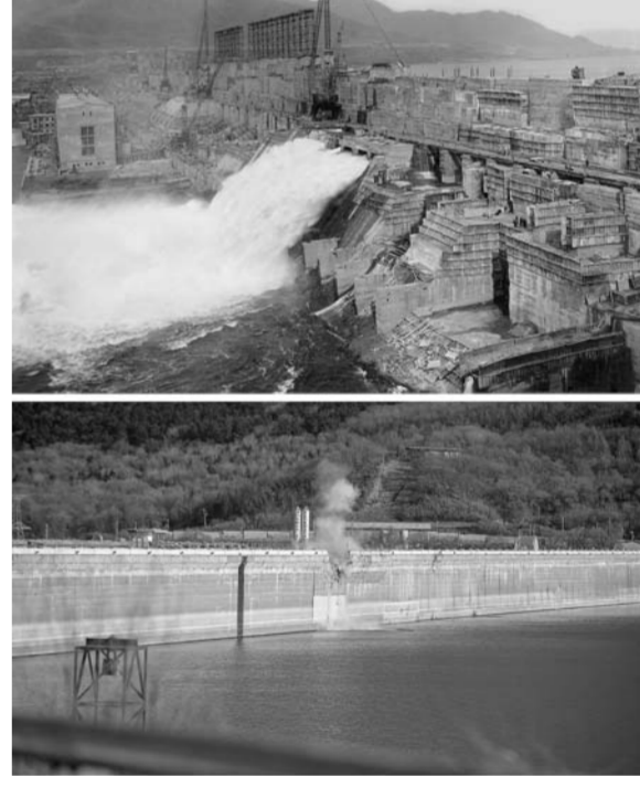
▲这是一张拼版照片。上图为1943年吉林市丰满大坝首台机组发电的景象(资料照片)，下图为丰满水电站原大坝爆破拆除工作现场(12月12日摄)。12月12日10时58分，随着一声巨响，位于吉林省吉林市松花江上的丰满水电站原大坝进入爆破拆除工序。丰满水电站是我国较早建成的大型水电站，被誉为“中国水电之母”，曾被印在1953年版的伍角人民币上。原大坝下游120米处，一座新坝已浇筑完工。
